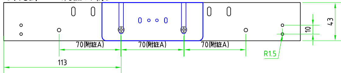
側視圖 -- 液晶面朝上
