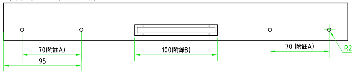
俯視圖 -- 液晶面朝上
