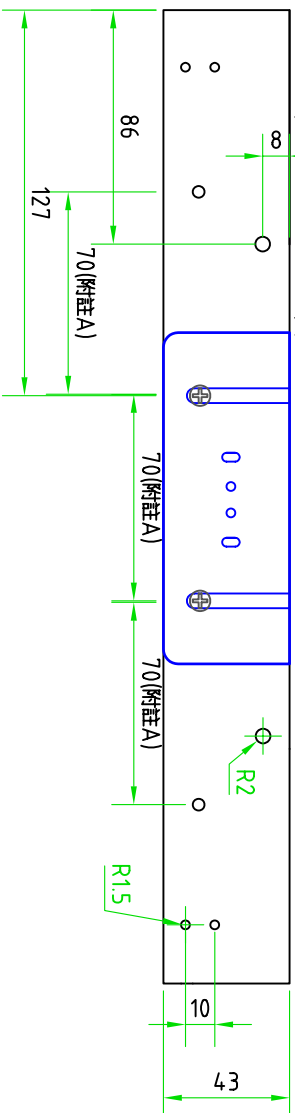
側視圖 -- 液晶面朝上
